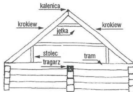
7a. Konstrukcja krokwiowa
