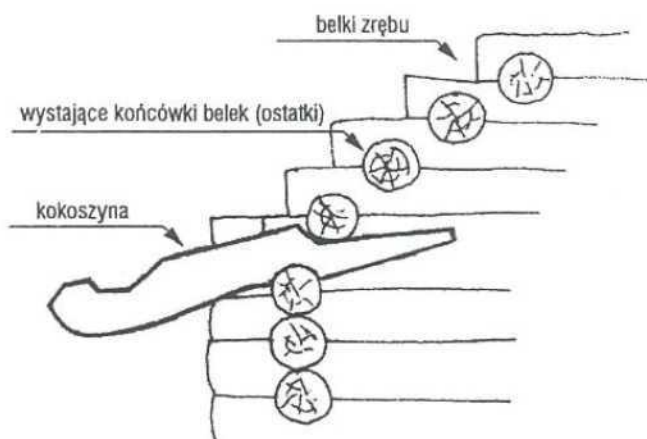
16. Kokoszyna – element konstr. ślegowej (b. archaiczny)
