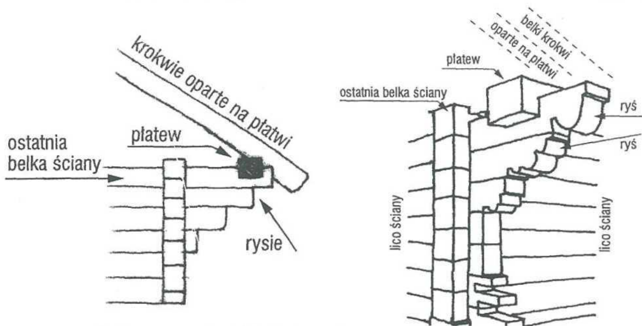
8. Konstrukcja krokwiowa z rysiami – krokwie oparte na płatwiach
