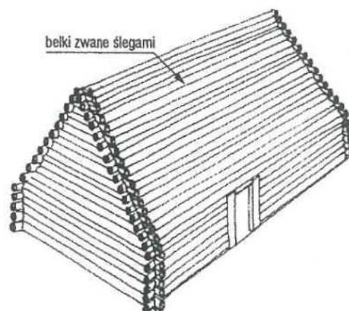
6. Konstrukcja ślegowa
