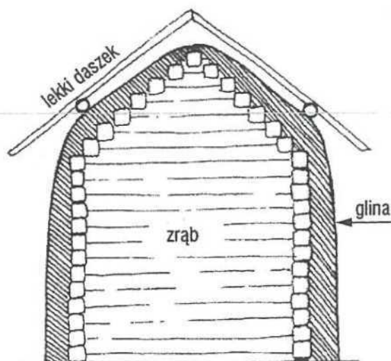
26. Sypaniec – przekrój
