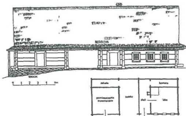
21. Chałupa łemkowska (Komańcza) – widok i plan
