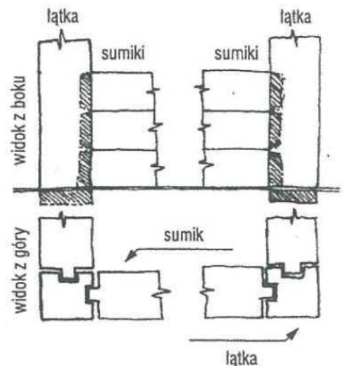
2. Wiązanie na rybi ogon
