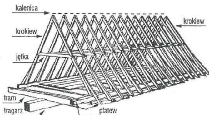
7b. Konstrukcja krokwiowa
