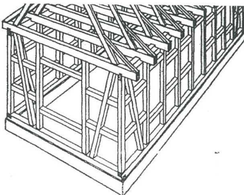
4a. Konstrukcja szkieletowa
