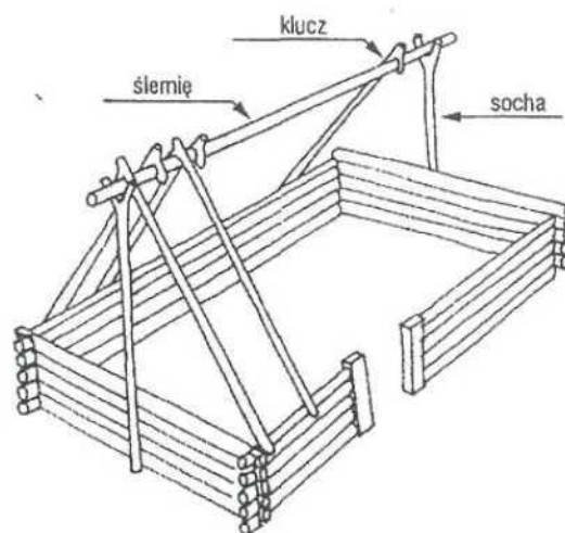
5. Konstrukcja sochowa
