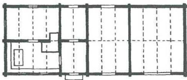
22. Chałupa łemkowska – plan
