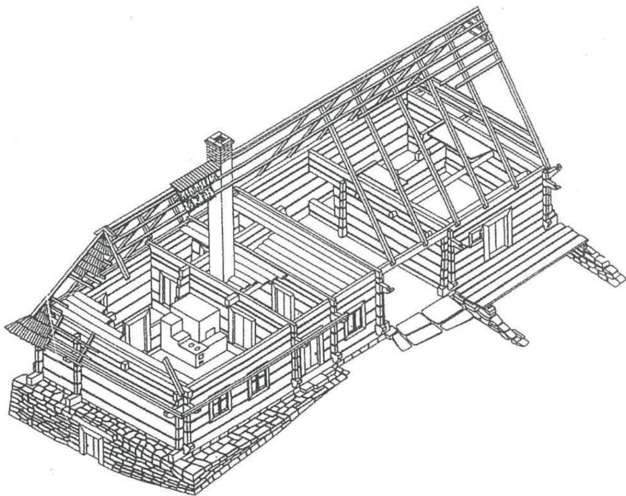
25. Chałupa łemkowska
