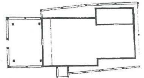
39. Dębno – plan
