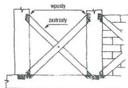
4b. Konstrukcja szkieletowa
