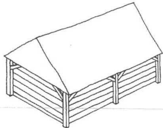
9. Konstrukcja przysłupowa
