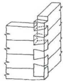
2. Wiązanie na rybi ogon
