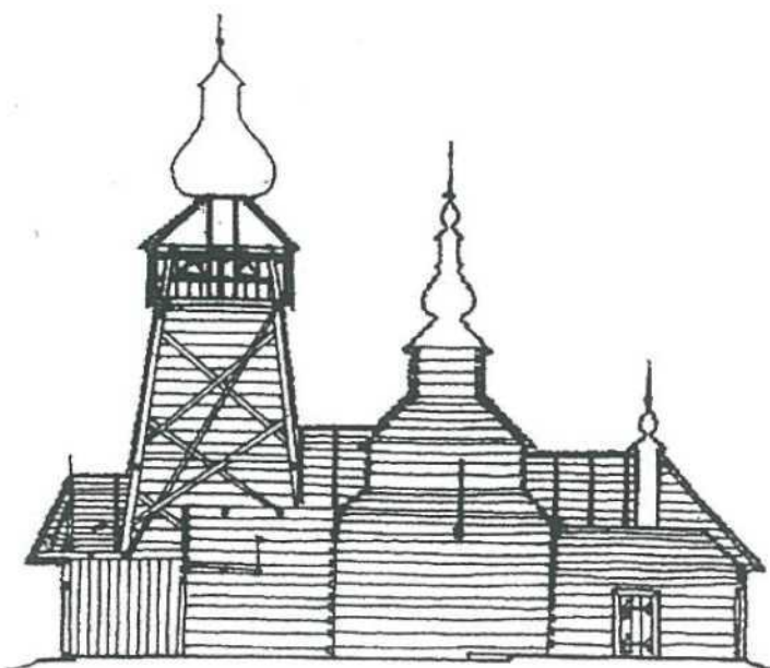
53. Cerkiew zachodniołemkowska (Powroźnik) – przekrój
