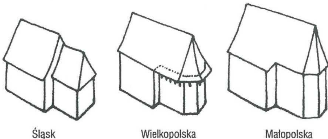
37. Układ więźby dachowej w kościołach poszczególnych grup
