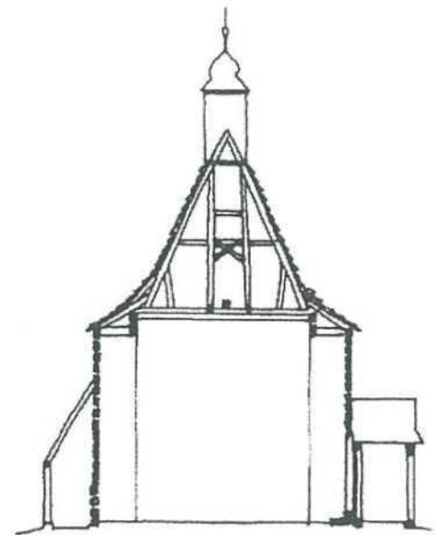
38. Dębno – przekrój
