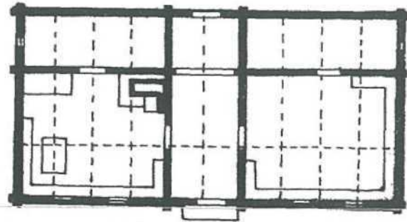
19. Chałupa podhalańska – plan
