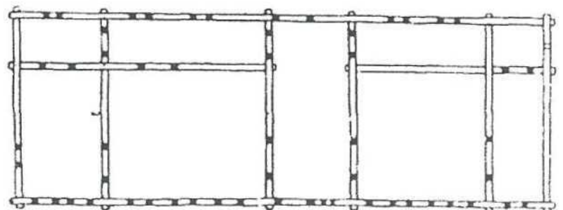
34. Dwór Moniaków (Zubrzyca G.) – widok i plan
